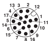
Polbild M12-Stecker, 17-polig, Ansicht Stiftseite
