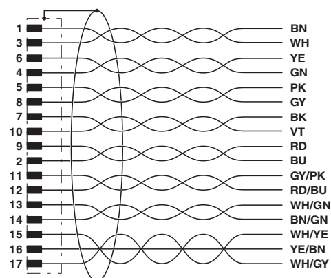
Kontaktbelegung des M12-Steckers
