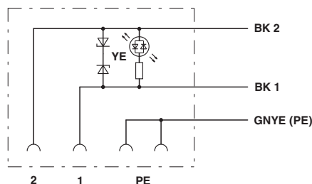
Schaltplan
