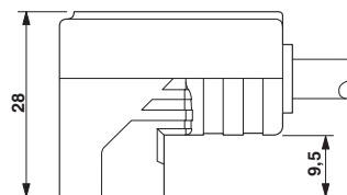
Ventilstecker, Bauform CI, Seitenansicht
