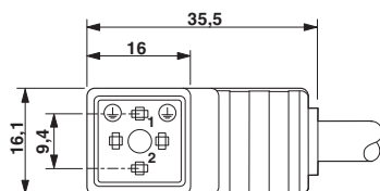
Ventilstecker, Bauform CI
