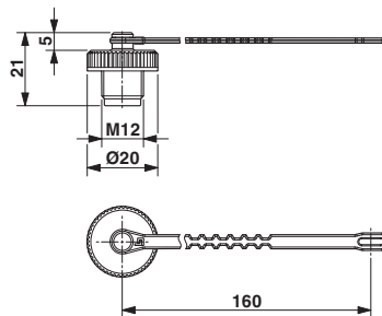
Maßzeichnung
