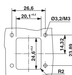
Maßzeichnung
