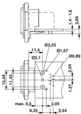
Bohrplan für VS-08-BU-RJ45/LP-1
