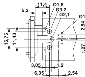
Bohrplan für VS-08-BU-RJ45-6/LH-1
