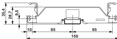
Maßzeichnung
