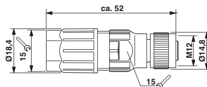
Maßzeichnung
