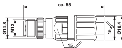
Maßzeichnung
