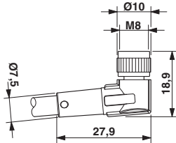
Maßzeichnung
