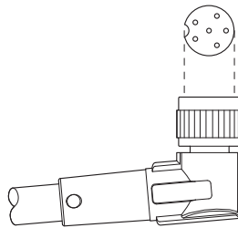
Schemazeichnung
