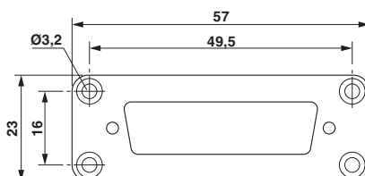
Maßzeichnung
