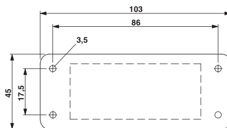
Maßzeichnung
