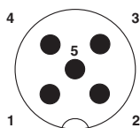
Pollbild M12-Stecker, 5-polig, A-kodiert, Ansicht Stiftseite
