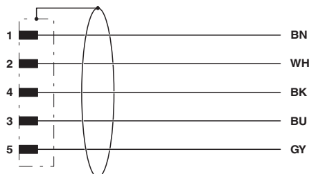
Schaltplan
