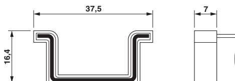
Maßzeichnung
