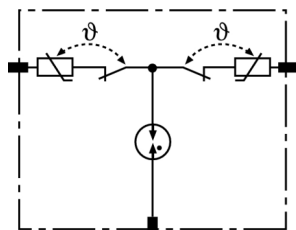
Prinzipschaltbild DR MOD 150
