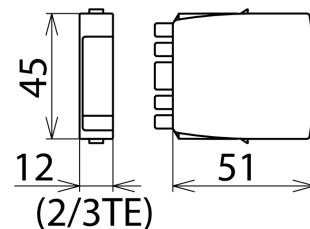
Maßbild BXT M4 T
