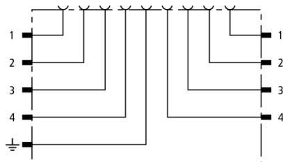
Prinzipialschaltbild BXT M4 T
