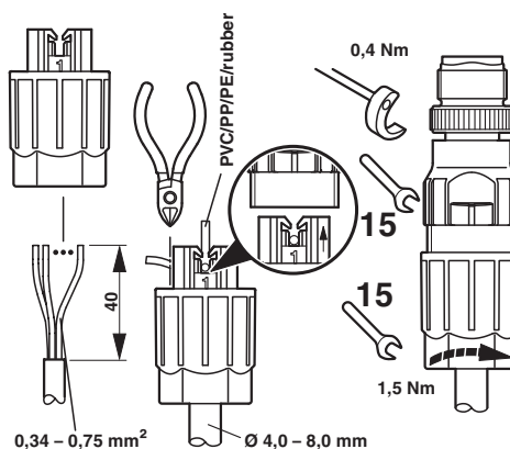
Maßzeichnung
