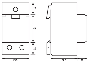
Maßzeichnung Gruppenansicht
