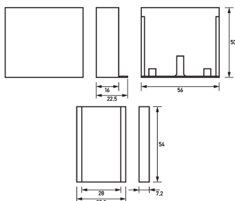
Maßzeichnung Gruppenansicht
