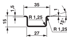
Maßzeichnung
