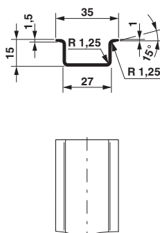
Maßzeichnung
