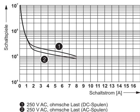
Elektrische Lebensdauer
