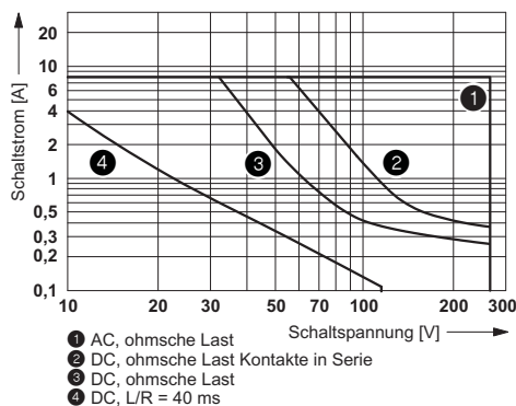
Abschaltleistung
