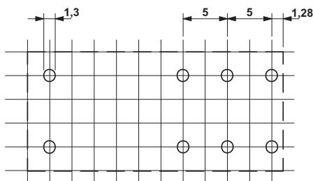
Bohrplan
