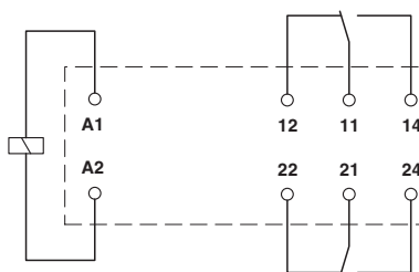
Schaltplan
