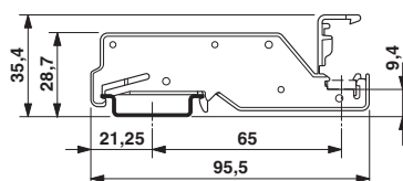
Maßzeichnung
