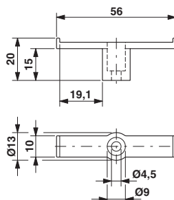
Maßzeichnung
