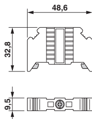
Maßzeichnung
