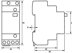
Maßzeichnung Gruppenansicht
