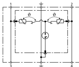
Prinzipialschaltbild DR M 2P 75
