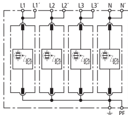
Prinzip Schaltbild DV M TNS 255
