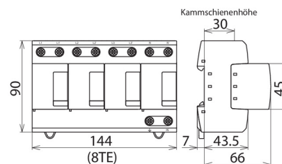
Maßbild DV M TNS 255
